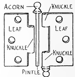
FIG. 447. BUTT HINGE.
